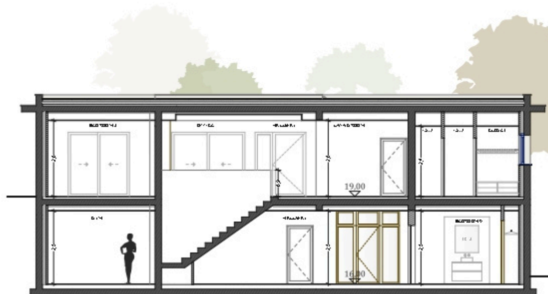
Corte BB'
