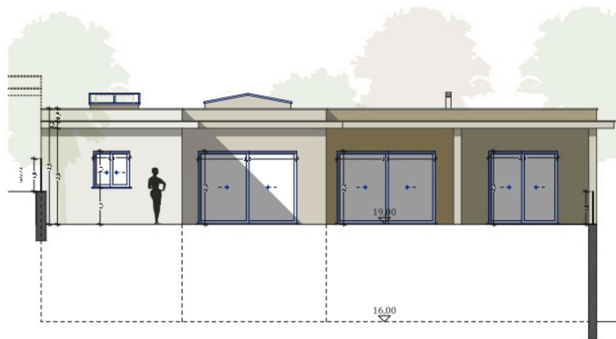
Alcado Este
