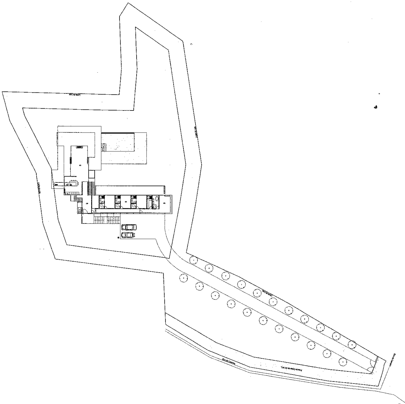
PLANTA DE IMPLANTAÇÃO Escala 1:250
